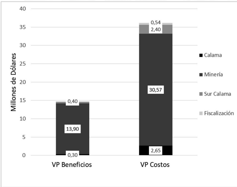
Figura 3: Reducciones en concentraciones del Plan por sector y medida
